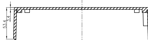
SECTION A-A
