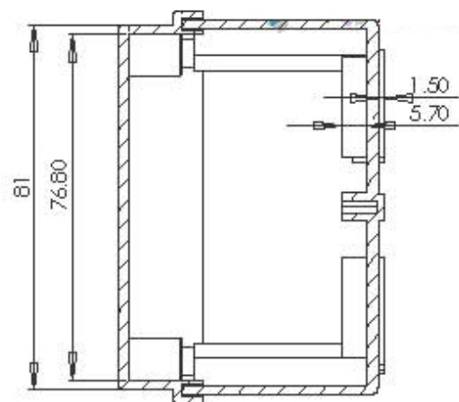
剖面 A-A
