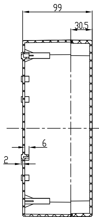
A-A
