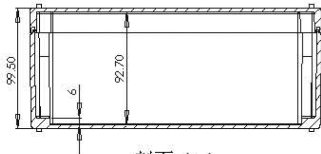
剖面 A-A
