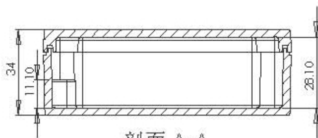
剖面 A-A
